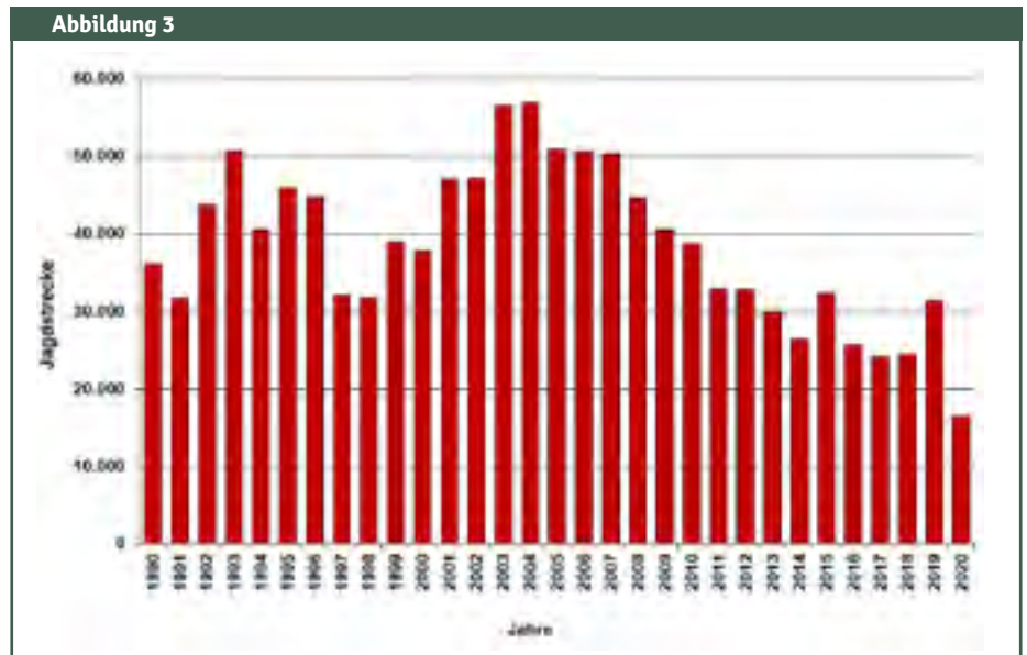
ABBILDUNG 3 | Entwicklung der Jagdstrecke des Feldhasen in Schleswig-Holstein im Zeitraum von 1990 bis 2020
