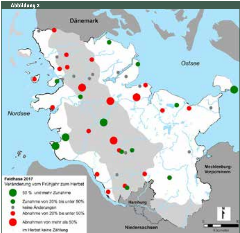
ABBILDUNG 2 | Der Sommerzuwachs des Feldhasen in Schleswig-Holstein im Jahr 2017
